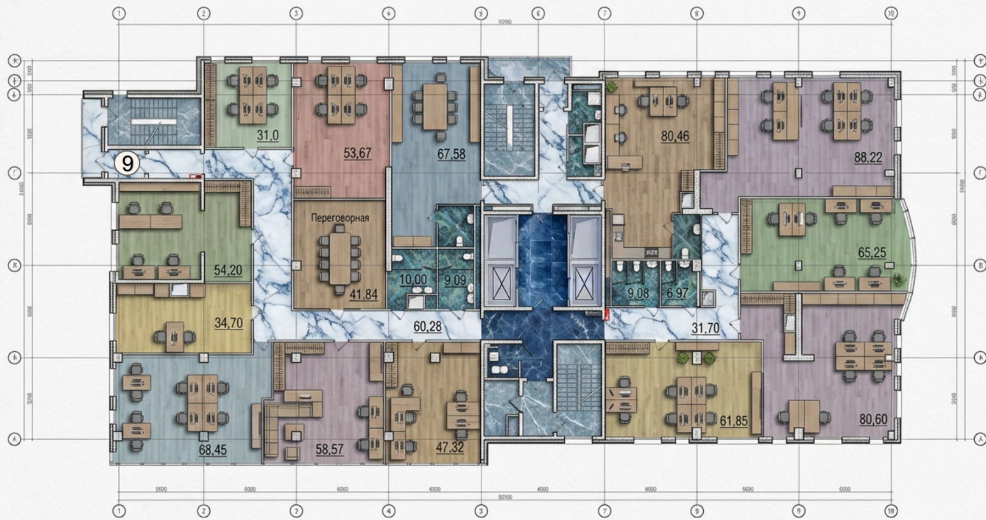
План 3-6 этажа
