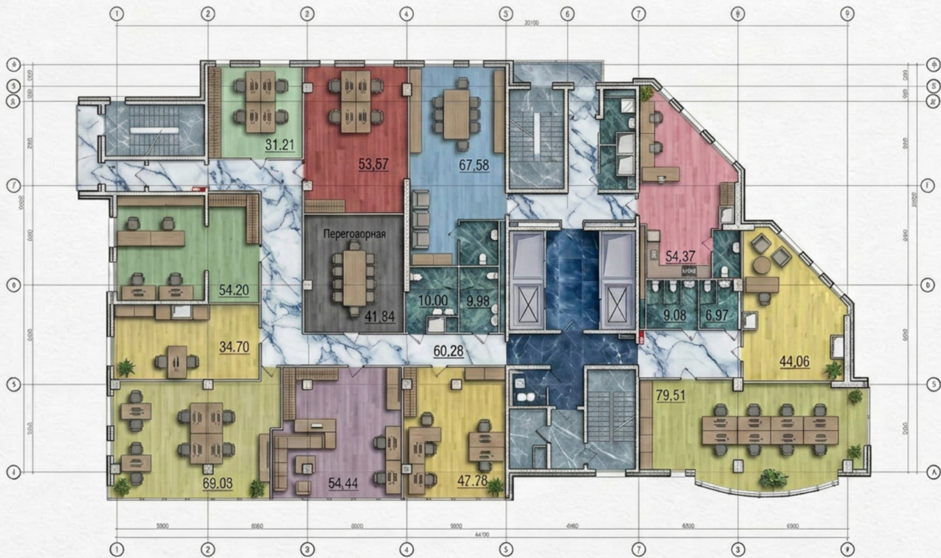
План 11 - 13 этажа
